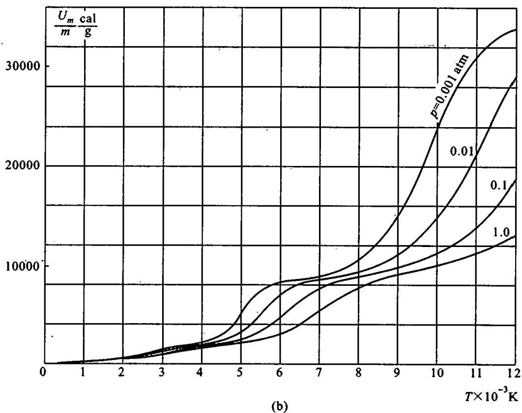
图 38. (a) 空气的热容对温度和压强的函数关系. 热容在温度高于 2000 K 时发生显著变化. (b) 空气的质量内能对温度和压强的函数关系
