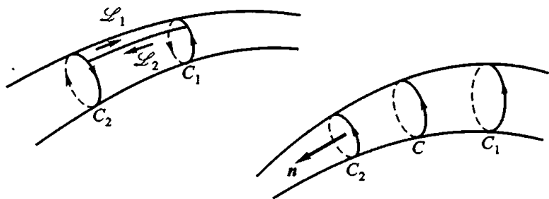
图 20. 用于研究涡管的性质
