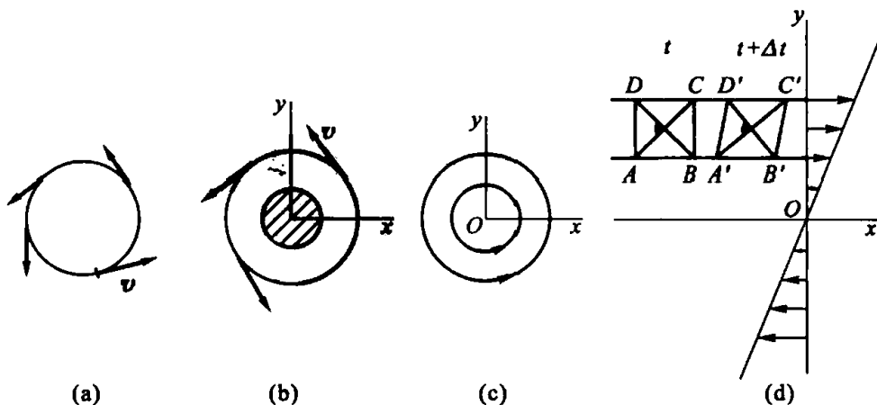
图 21. 可能出现的有旋流动与无旋流动的例子
