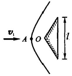
图 59. 在绕大顶角楔形物体的流动中, 在有限物体前方某处形成激波
