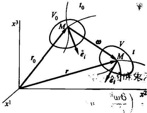
图 12. 位移矢量
