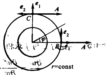
图 13. 平面上的极坐标系
