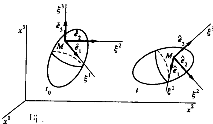
图 10. 刚体的运动
