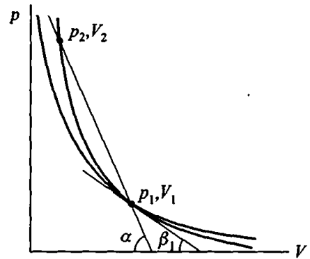
图 51. \beta_1 是泊松绝热线的切线与 V 轴形成的锐角, \alpha 是于戈尼奥绝热线的割线与 V 轴形成的锐角
