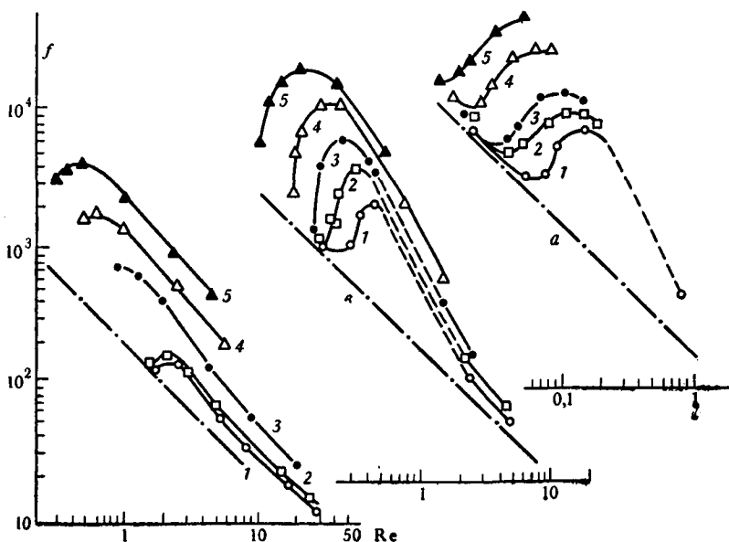
РИС. 20. Зависимость f(Re) для раствора полиоксипропилена WSR-301. Концентрация полимера:
