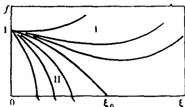
РИС. 10. Интегральные кривые уравнения (II.153)
