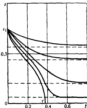
РИС. 47. Распределение насыщенности при противоточной капиллярной пропитке
