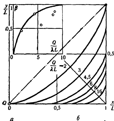
РИС. 54. Расположение целиков и зависимость коэффициента охвата для пятиточечной схемы площадного заводнения от интенсивности потока
