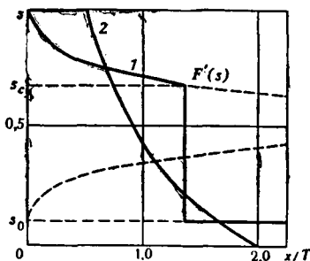
РИС. 40. Распределение насыщенности при автомодельном решении задачи Баклея — Леверетта: 1 — для проницаемостей, показанных на рис. 37; 2 — для прямолинейных относительных проницаемостей ( \mu_0 = 0,5 )
