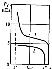
РИС. 36. Кривые капиллярного давления (насыпная среда проницаемостью 7 мк/м²):
