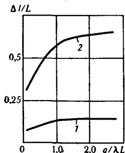
РИС. 27. Зависимость ширины трубки тока от интенсивности потока q/\lambda L при фильтрации с предельным градиентом. Расход через квадратный элемент пятиточечной сетки в %:
